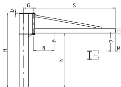
Gru a colonna Rotazione 300°
